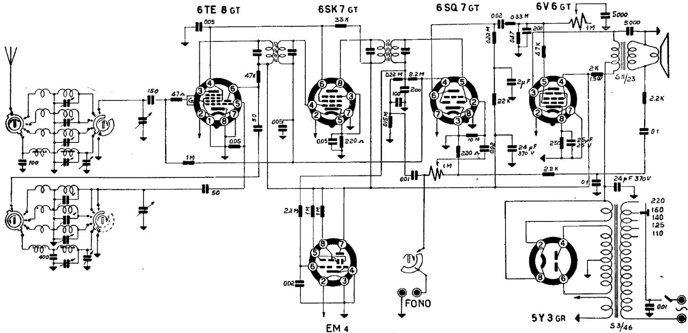
MINERVA RADIO - Mod. PORTOVENERE 535/3. Supereterodina a 5 valvole. Quattro gamme d'onda: onde medie da 109 a 580 m; onde corte da 15,5 a 22,5 m, da 22 a 35,5 m, da 33 a 52 m. Media frequenza 468 kc/s. Potenza d'uscita 3,5 watt. Consumo 40 watt.
